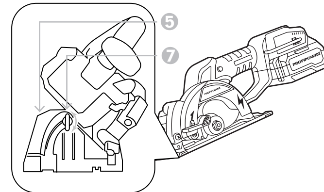
Рисунок 2.1.4. Установка угла наклона основания
