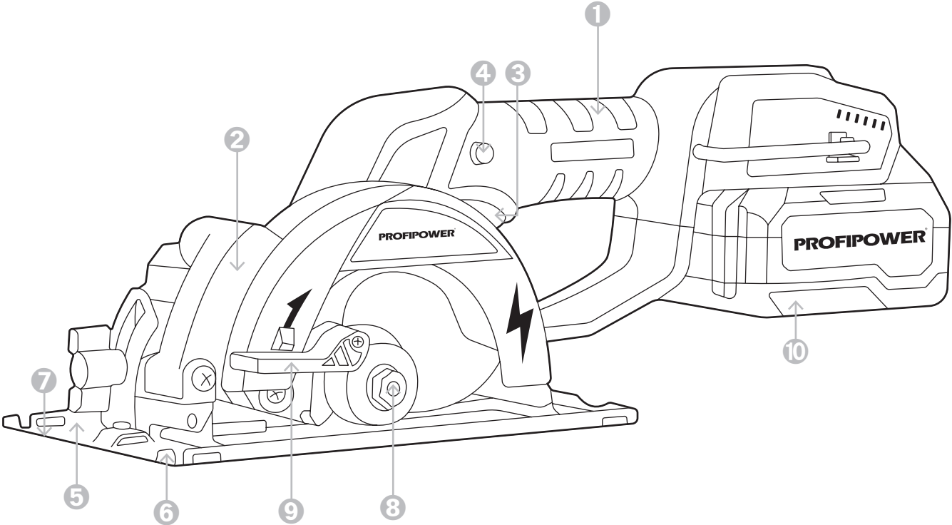
Рисунок 1.4.1. Устройство инструмента
